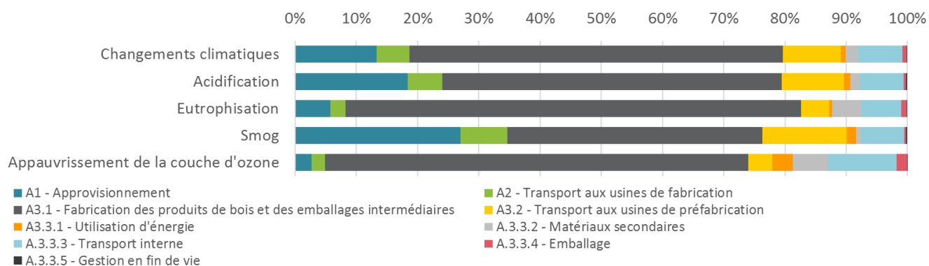
Figure 2: Contribution relative des principaux procédés de production des poutrelles de plancher
