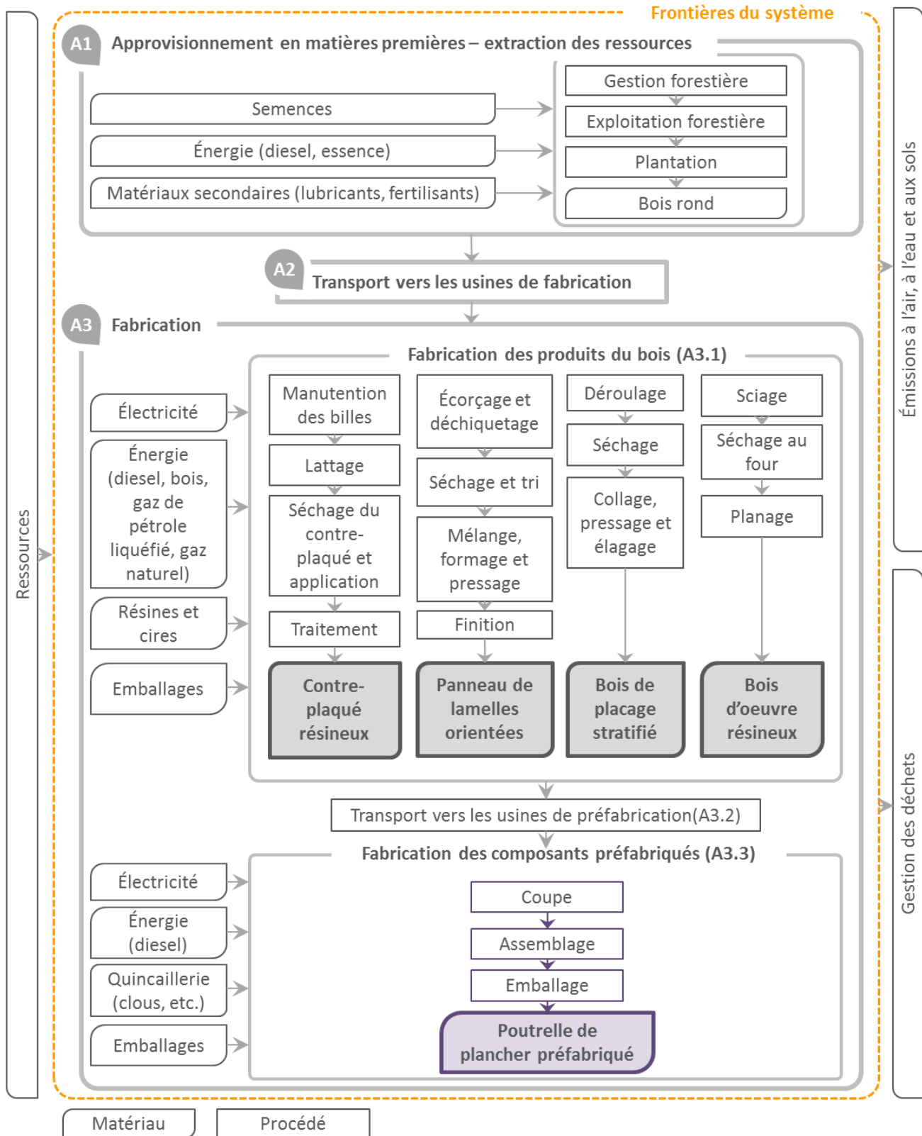
Figure 1: Procédé de fabrication des poutrelles de plancher
